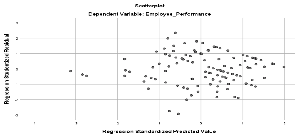
Gambar 1. Grafik Scatterplot
